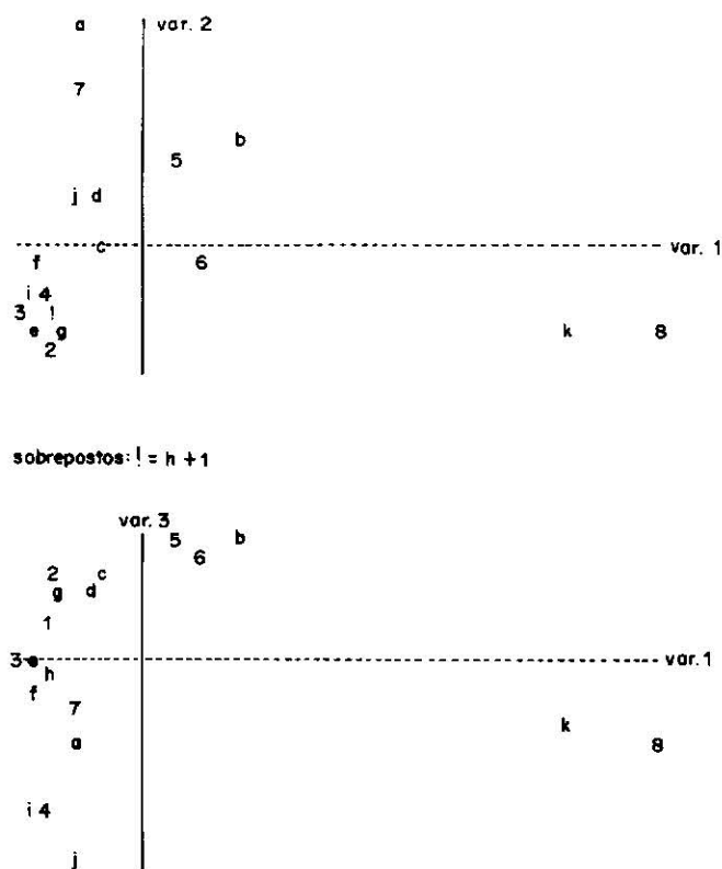
FIG. 1. Dispersão das três principais variáveis canônicas geradas na análise de concentração da Tabela 2. Os pontos estão identificados pelos respectivos grupos de quadrados (1-8) ou de espécies (a-k).
