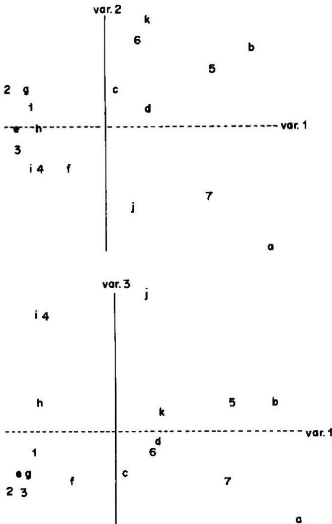
FIG. 2. Dispersão das três principais variáveis canônicas geradas na análise de concentração da Tabela 2, excluindo-se o grupo 8 ( Eleocharis-Centella ). Os pontos estão identificados pelos respectivos grupos de quadrados (1-7) ou de espécies (a-k).
